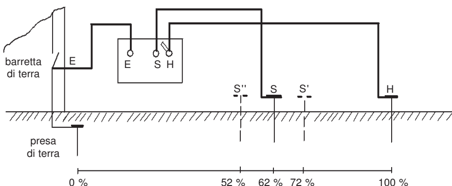
Misura di resistenza di una presa di terra con il metodo del 62%
