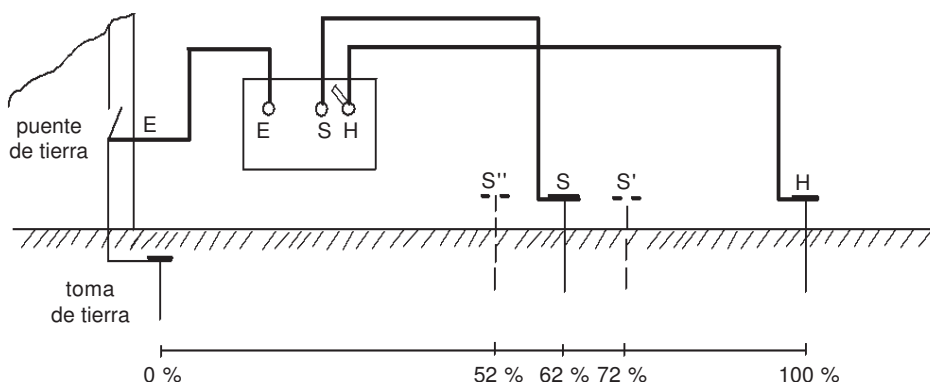
Medida de resistencia de tierra mediante el método del 62%.
