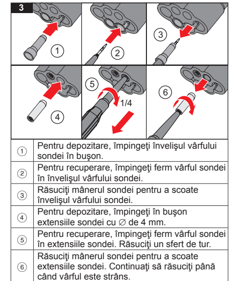
Figura 3 ilustrează modul în care trebuie depozitate și recuperate accesoriile de vârf din bușon.
