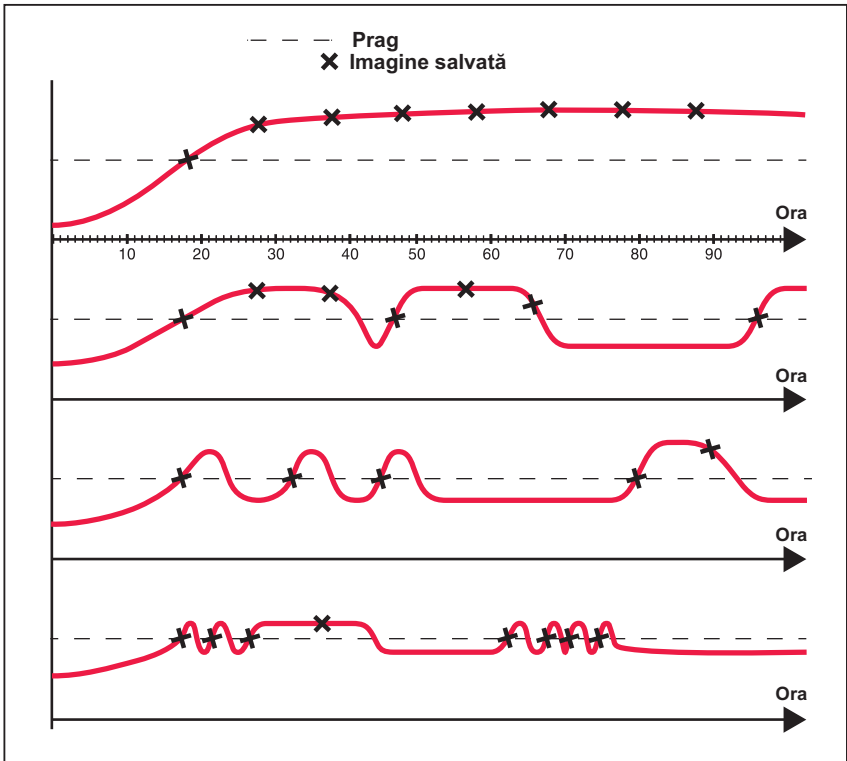
Figura 11. Scenarii de capturare a imaginilor pentru Alarma de monitorizare automată
