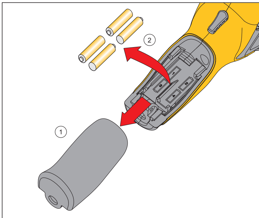
Figura 12. Înlocuirea bateriei VT02, VT04A
