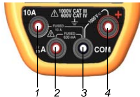
Figure 4 : les bornes
