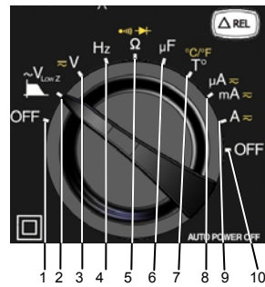
Figura 1 : el conmutador
