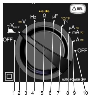
Figura 1 : il commutatore
