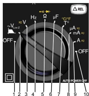
Abbildung 1 : Drehschalter
