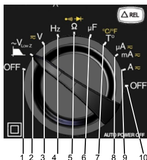
Figure 1 : le commutateur
