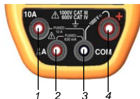
Abbildung 4 : die Buchsen
