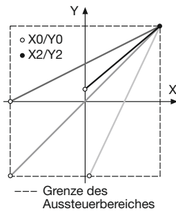
Bild 8. Beispiele für Einstellmöglichkeiten bei linearer Kennlinie.
