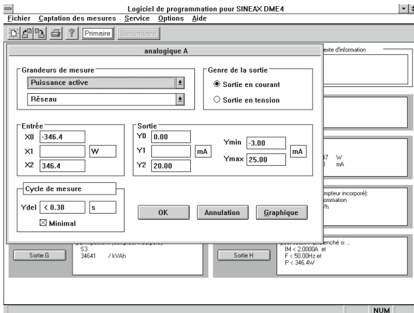
Fig. 11. Programmation des grandeurs de sortie.
