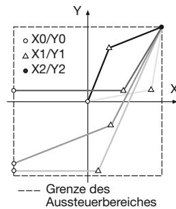
Bild 9. Beispiele für Einstellmöglichkeiten bei geknickter Kennlinie.
