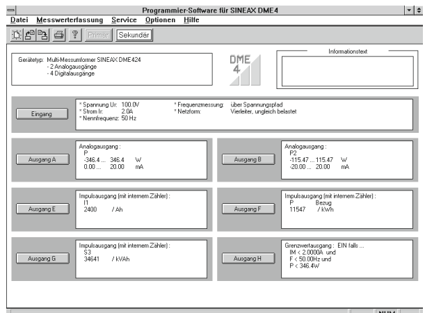
Bild 10. Darstellung aller Programmierparameter im Hauptmenü.
