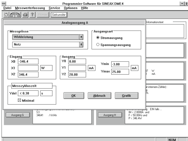
Bild 11. Programmierung der Ausgangs-Messgrößen.
